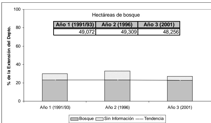
Figura: Comparación de la cobertura forestal de Quetzaltenango en los 3 períodos
